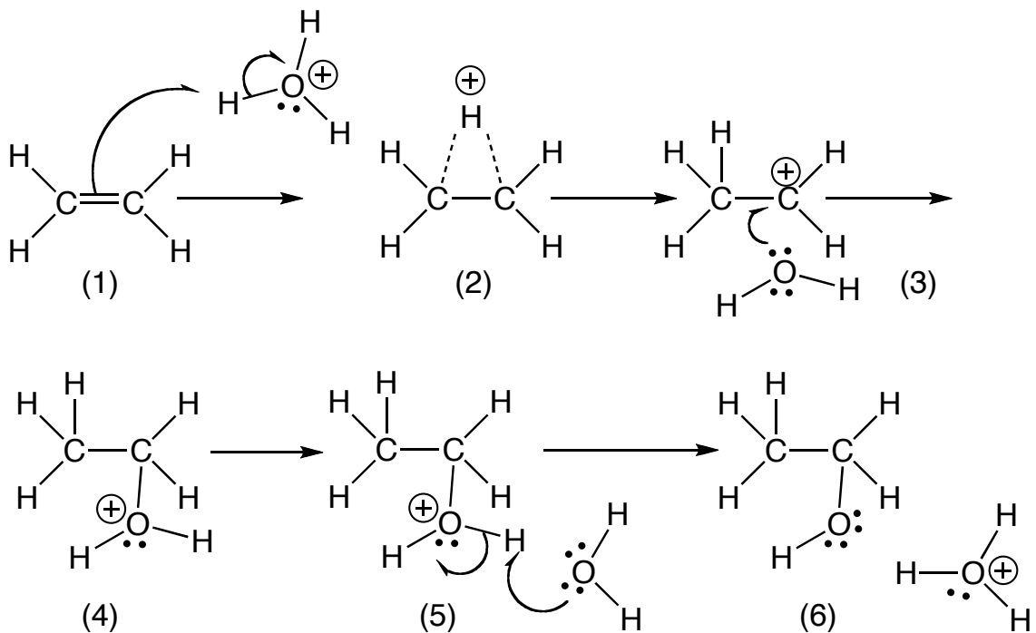
図 3 エチレンへの水の付加反応。(1) \pi 電子が \text{H}_3\text{O}^+ に引き寄せられる。(2) C-C 結合上部で \text{H}^+ がつかまった状態になる。(3) H 原子をつかまえてなかった C 原子には + 電荷が移る。ここを \text{H}_2\text{O} の非共有電子対が攻撃する。(4) 水分子がつかまり、+ 電荷は O 原子に移る。(5) ここから別の \text{H}_2\text{O} が塩基として働いて \text{H}^+ を引き抜いて行く。(6) \text{H}_3\text{O}^+ が再生される。これは再び(1)の反応に用いられる。
