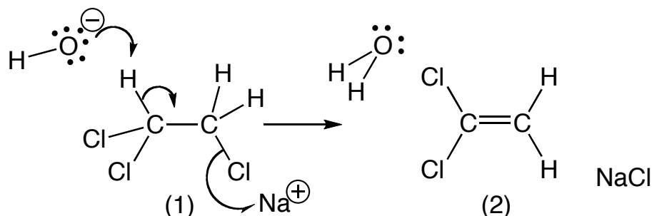
図 5 1,1,2-トリクロロエタンからの脱離反応による塩化ビニリデンの生成. (1) \text{NaOH} からの \text{OH}^- が水素原子を攻撃し、 \text{H}^+ を引き抜こうとする. 同時に、 \text{NaOH} からの \text{Na}^+ が隣の \text{C} 原子から \text{Cl}^- を引っ張る. (2) \text{H}^+ と \text{Cl}^- はそれぞれの \text{C} 原子から離れて行き、同時に 2 個の \text{C} 間に二重結合が生じ、アルケンとなる.
