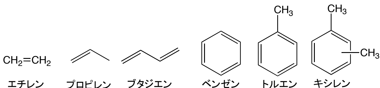
図7 石油化学基礎製品. ここでキシレンは3種類の異性体( o -キシレン, m -キシレン, p -キシレン)を一括して描いてある。
