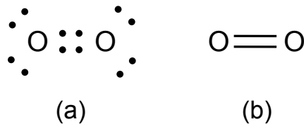
図 12 酸素分子 O 2 の構造. (a)点電子図, (b)結合図.
