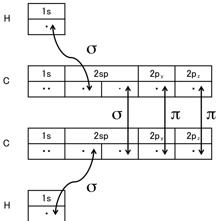
図 19 アセチレン分子 \text{CH}\equiv\text{CH} を構成する 4 個の原子それぞれにおける電子配置と, 共有結合の生成.
