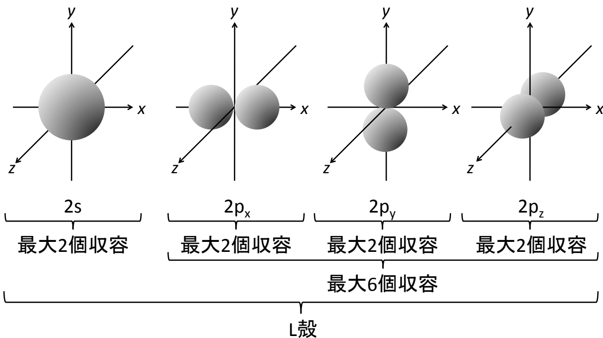
図4 L殻の原子軌道。2s、 2p_x 、 2p_y 、 2p_z の4軌道から構成される。 2p_x 、 2p_y 、 2p_z は等価な軌道だが、これら3軌道と2s軌道とは等価ではない。 2p_x 軌道の場合、y-z平面以外の全空間、が電子の存在し得る空間である。同様に 2p_y 軌道の場合にはz-x平面以外の全空間、 2p_z 軌道の場合にはx-y平面以外の全空間に電子が存在可能である。いずれも「だいたいこのあたりに電子が見つかる」と考えて良い」空間のイメージはこの図のようになる。
